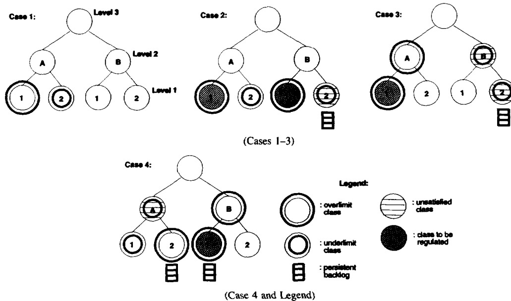
Fig. 4. Examples of link-sharing scenarios.
